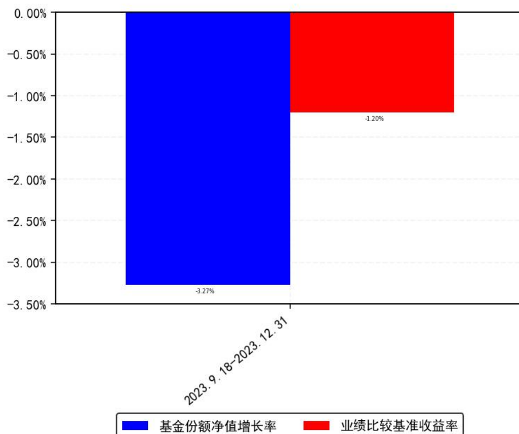
招商安瑞进取债券C每年净值增长率与同期业绩比较基准收益率的对比图
